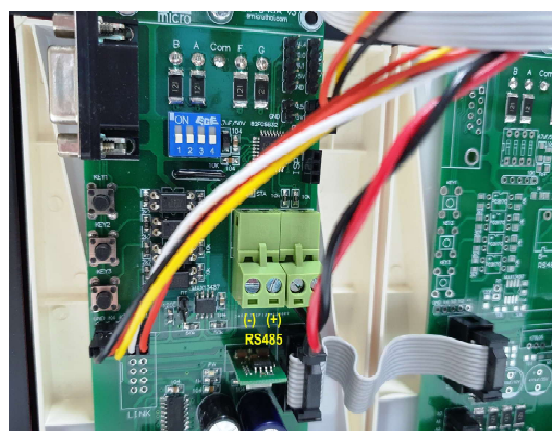
ขั้วต่อ RS485 และ Dip-Switch
