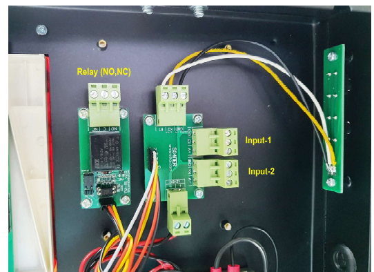
ขั้วต่อ Input และ Relay
